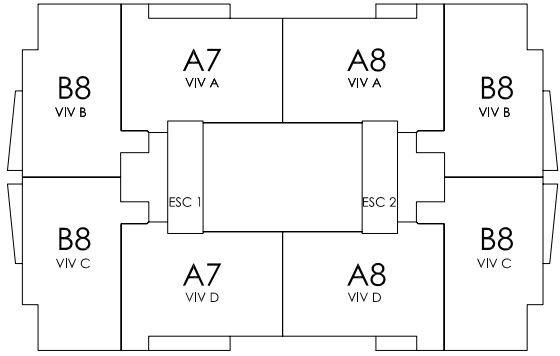
PLANTA 8ª
